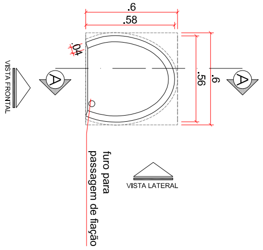
Planta Baixa - Púlpito ESC.: 1/25
