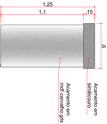
Vista Lateral - Púlpito ESC.: 1/25
