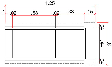
Vista Frontal - Púlpito ESC.: 1/25
