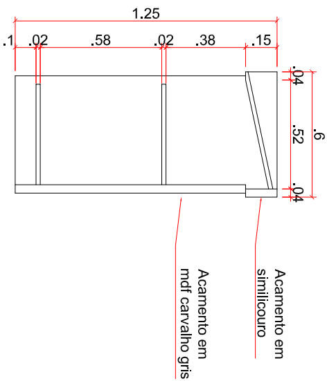
Corte AA - Púlpito ESC.: 1/25
