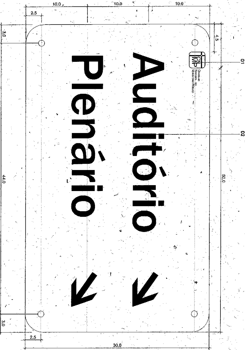
VISTA FRONTAL UNIDADE: cm
